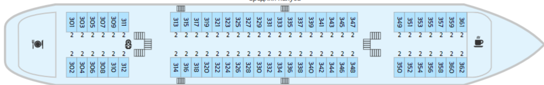
Главная палуба
